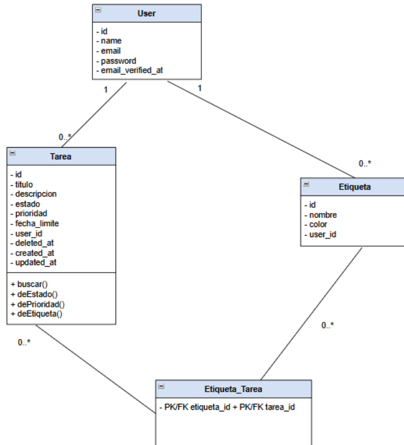
Figura 3. Modelo de datos con tabla pivote. Fuente: Elaboración propia a partir de modelos y migraciones.
