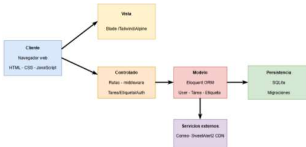
Figura 1. Arquitectura lógica MVC implementada. Fuente: Elaboración propia a partir del código auditado.
